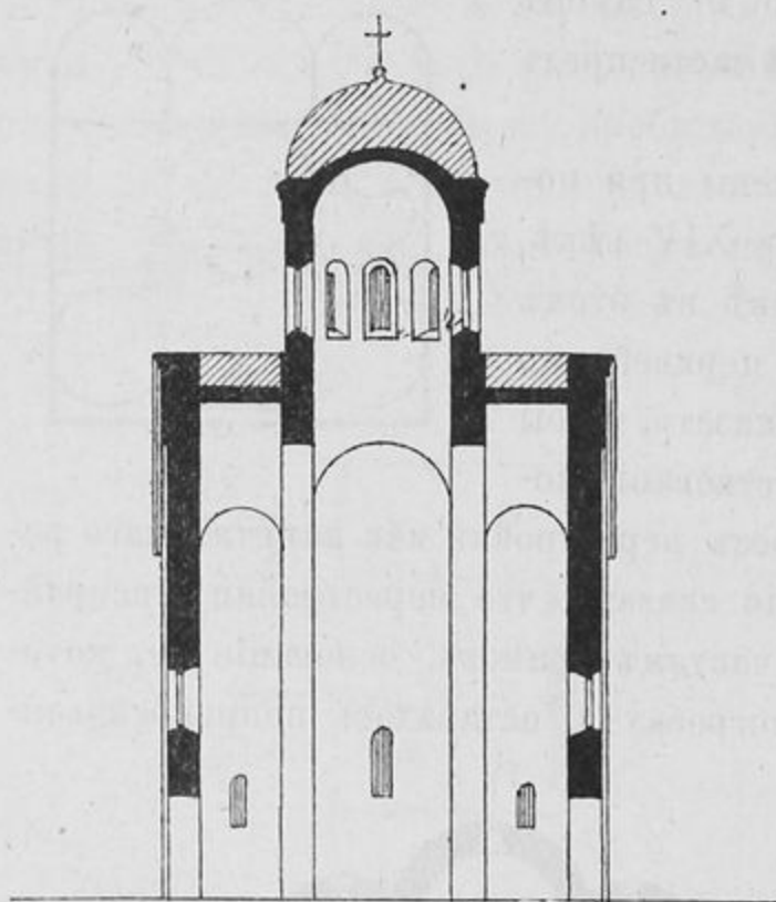
Разрѣзь по линіи АВ.
